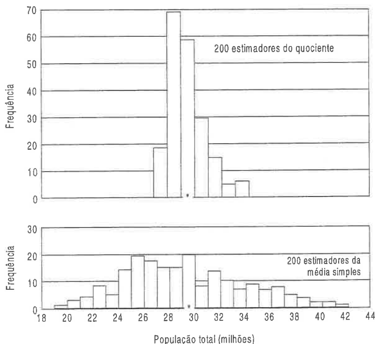
Figura: Comparação experimental do estimador do quociente com o estimador baseado na média da amostra.
