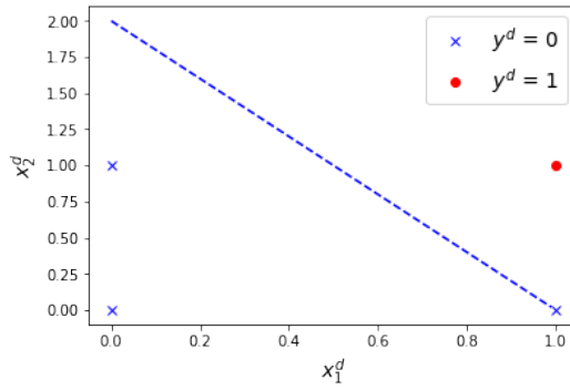
Figura 6.10: A fronteira de decisão do Perceptrão
